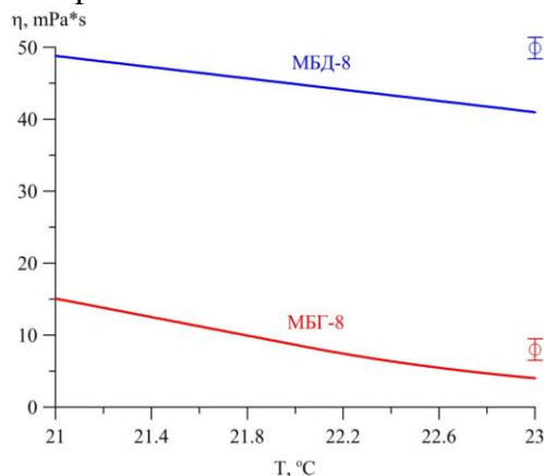
6 сурет – Турбина майлары тұтқырлығының температурадан тәуелділігі
