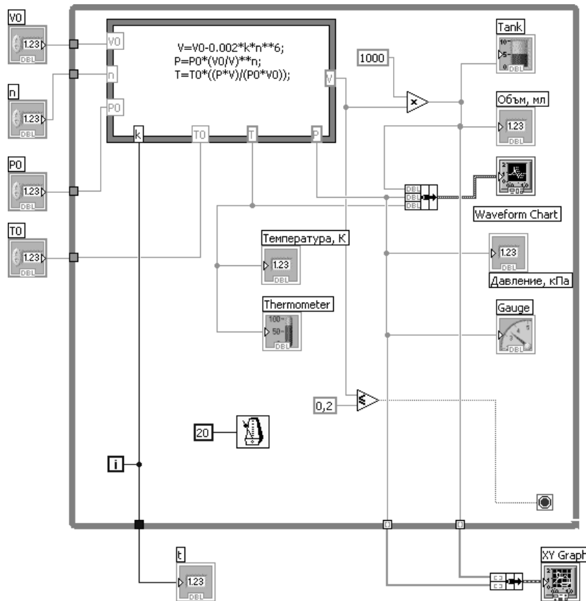
Рисунок 2 - Блок-схема программы расчета
